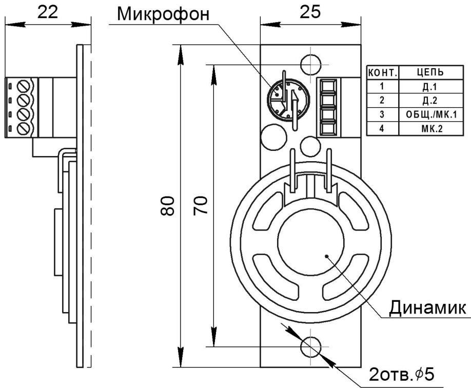
Рис.1 Внешний вид Платы громкоговорящей связи ПГС-МД НШЕК.465319.005
